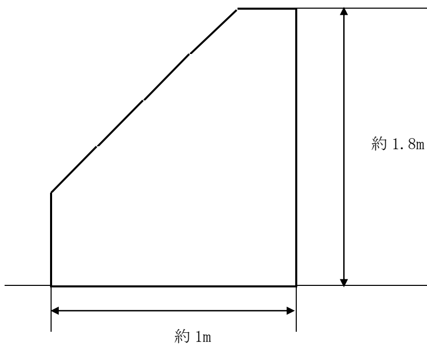
祭壇（横断面）
