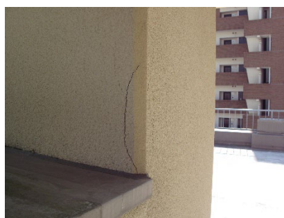
庁舎別館 外壁：D 仕上げ材の割れ
