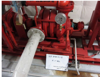
保健センター 防災消防設備：D 消防ポンプの漏水
