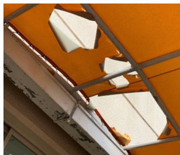
上野口保育園 窓・扉（外部）：D ガラスの割れ
