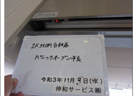
保健センター 窓・扉（外部）：A 自動扉パニックオープン不良
