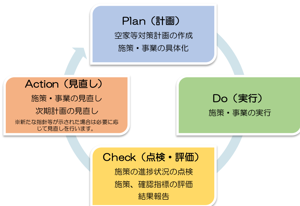
図8-2 PDCA サイクル
