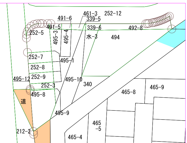
大図 7
