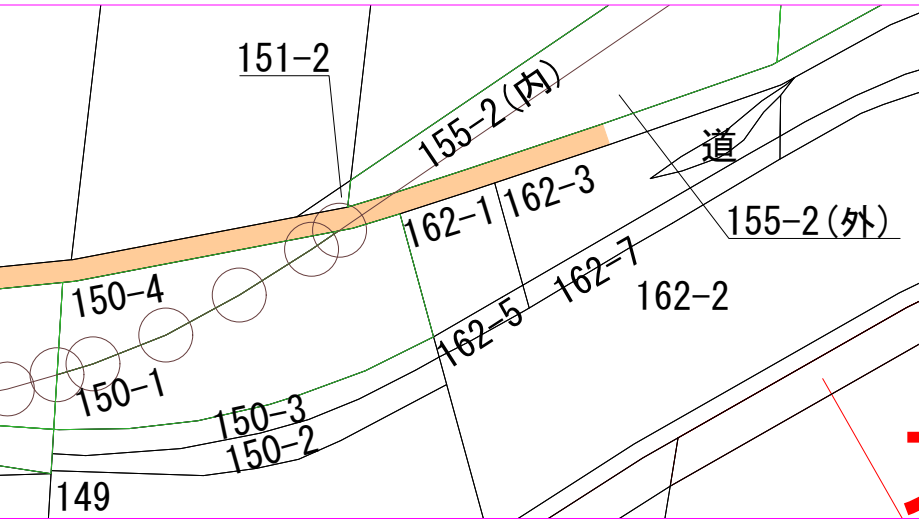
拡大図 5
