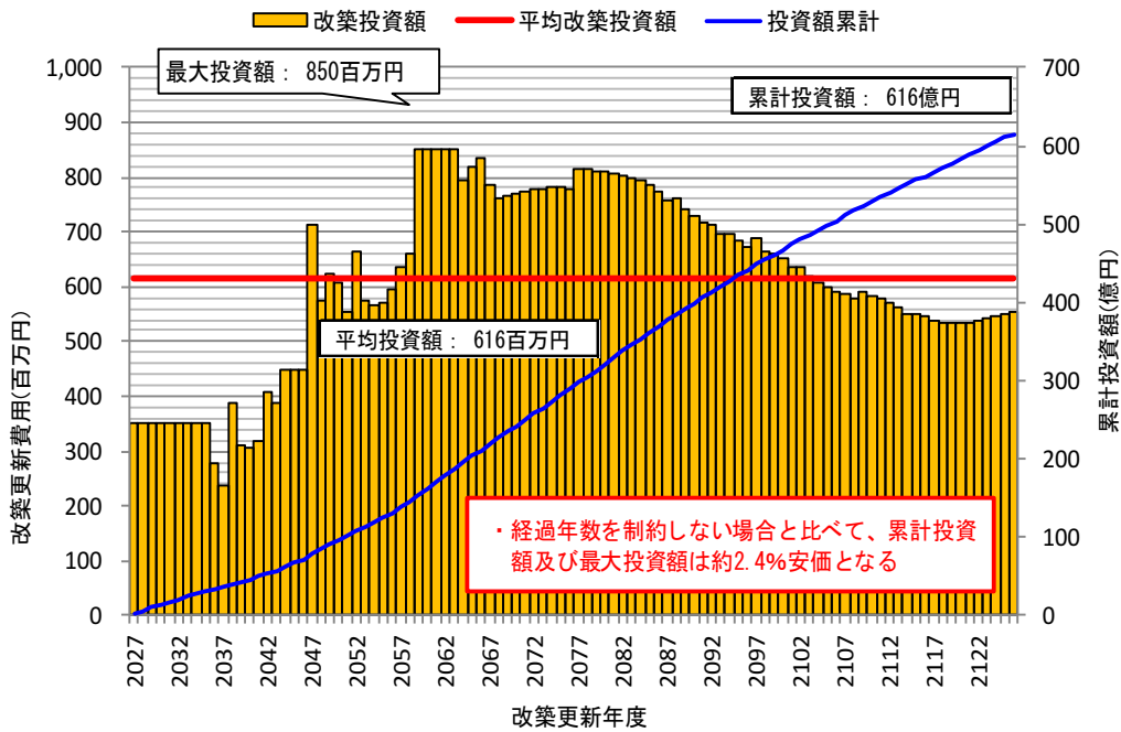
図 1-4 パターンVIの事業費予測
