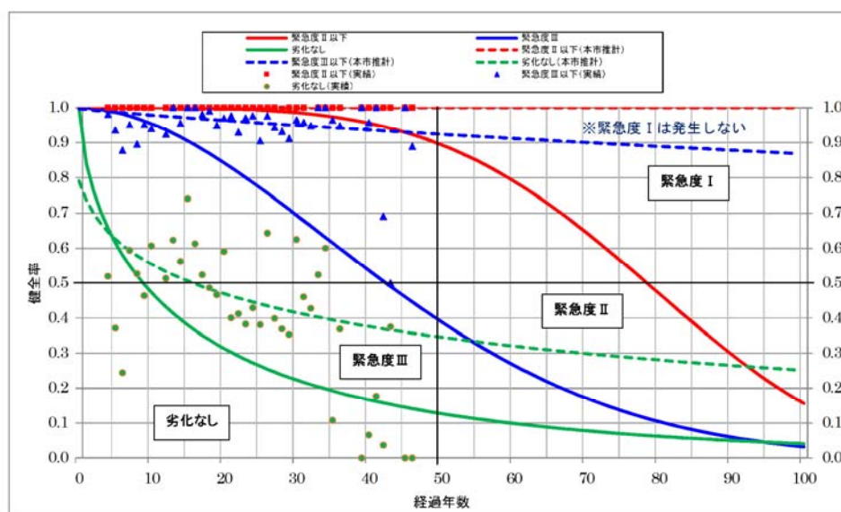
図 1-3 本市が独自作成した健全度予測式
