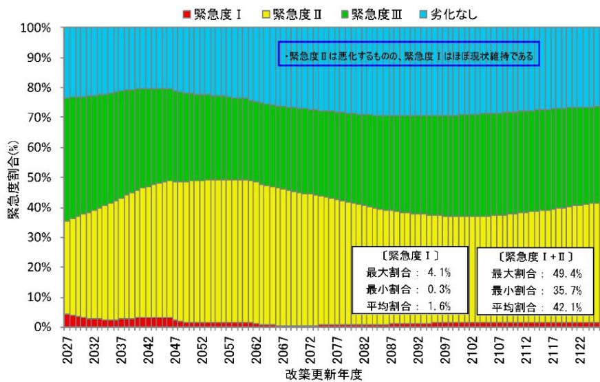
図 1-5 パターンVIの健全度予測
