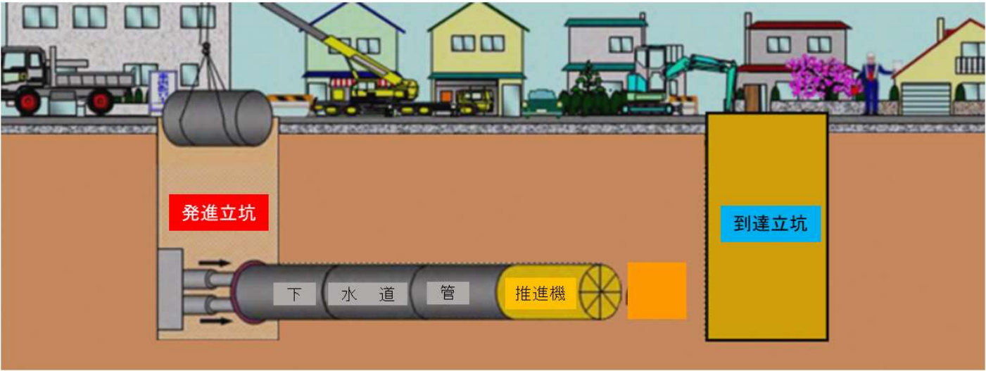
推進工法の作業イメージ
