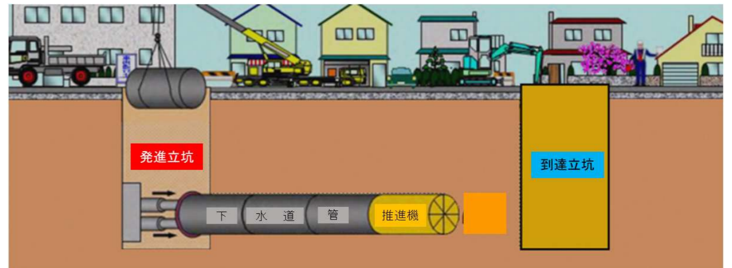
推進工法の作業イメージ
