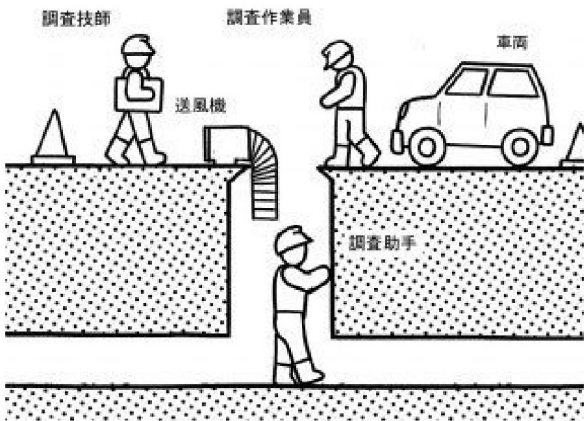
作業様式図
