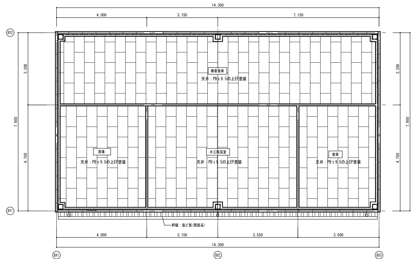
市民プラザ別棟2 天井伏図 1 : 50
