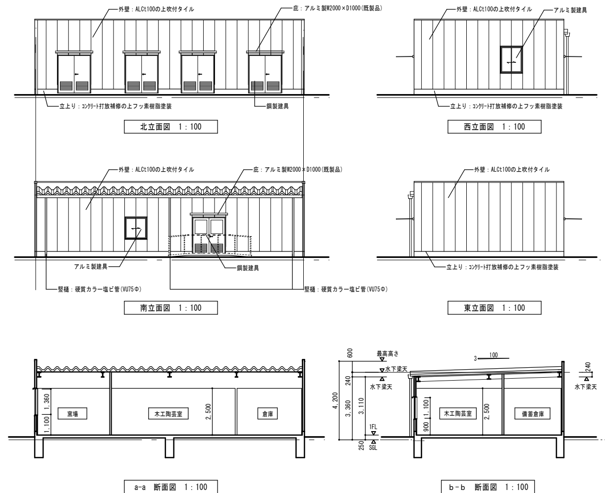
b-b 断面图 1:100
