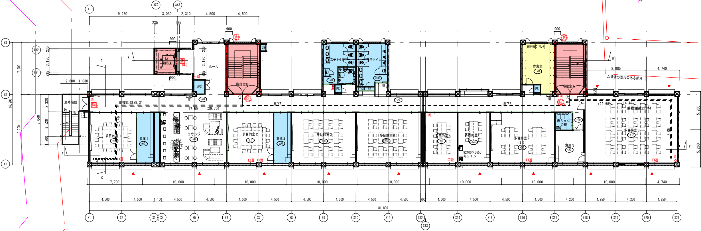
3階平面図 1:150
