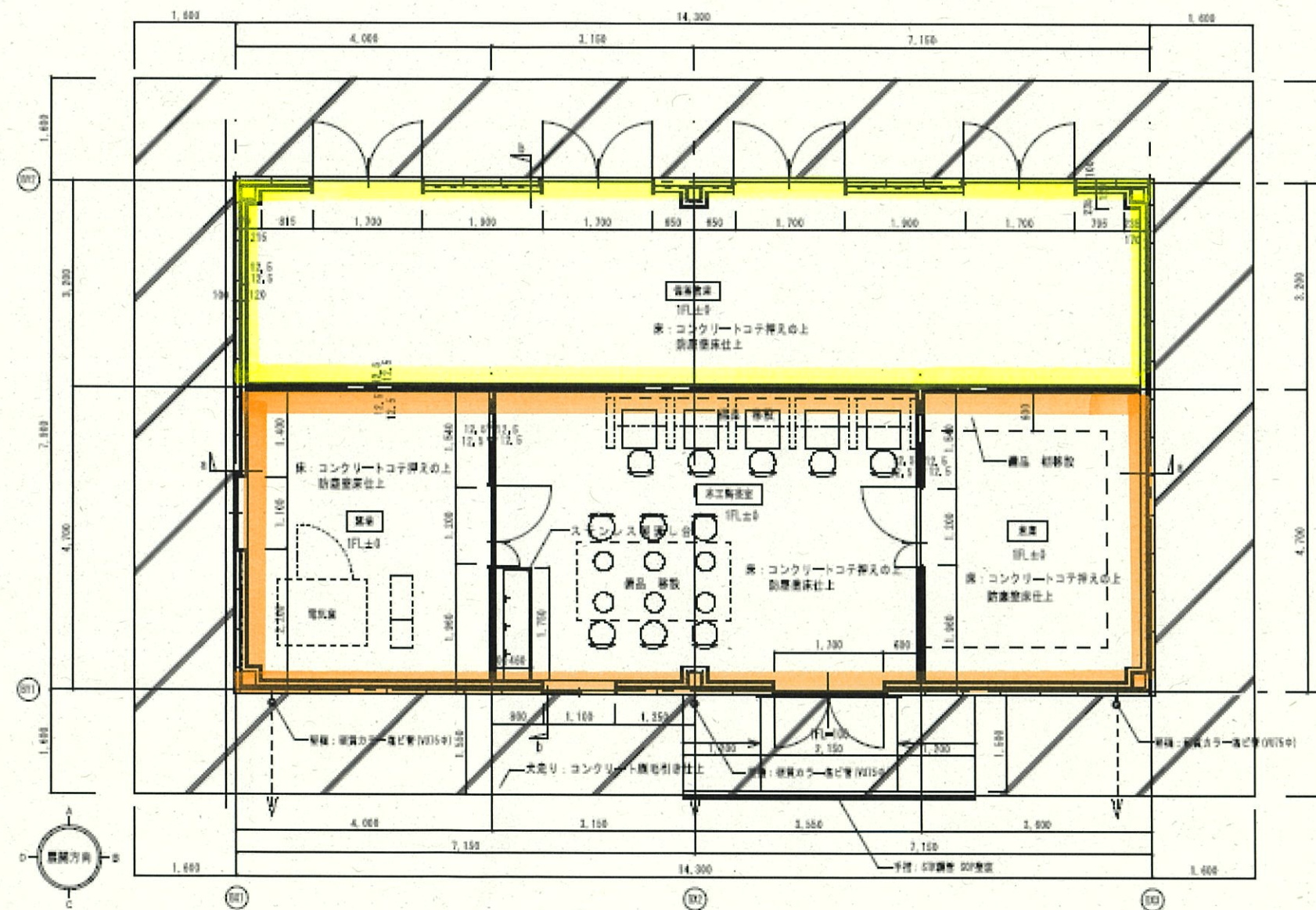
新市民プラザ 別棟2
