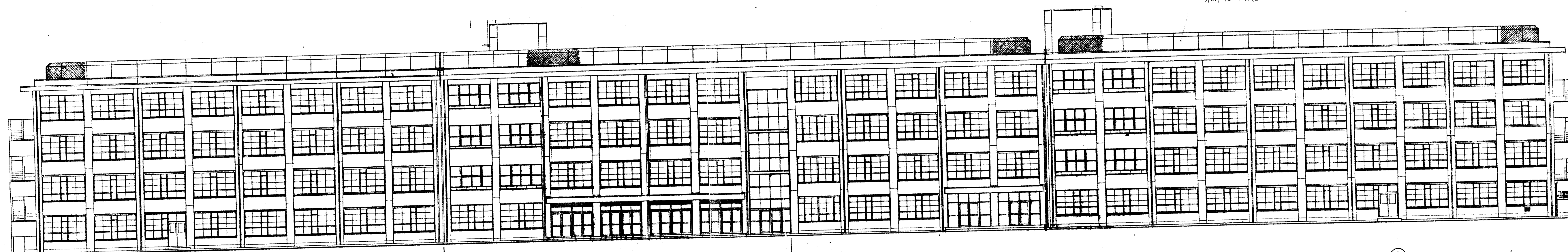
③ 立面图 1/200
