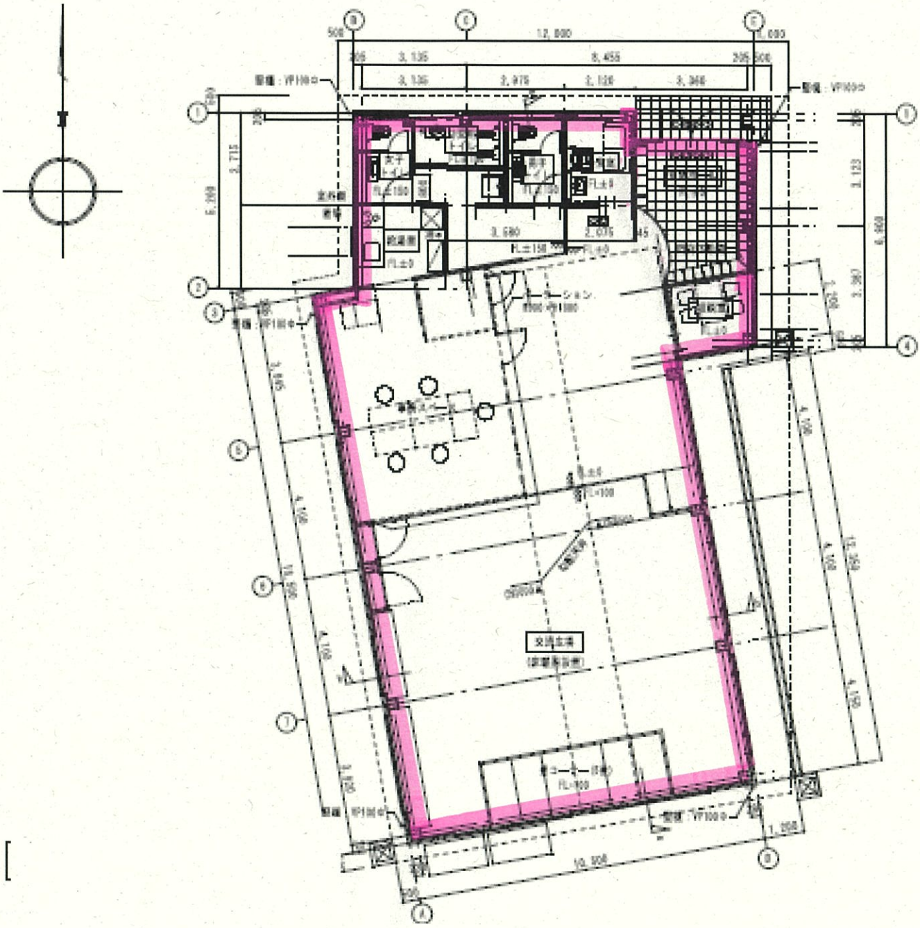
新市民プラザ 別棟1
