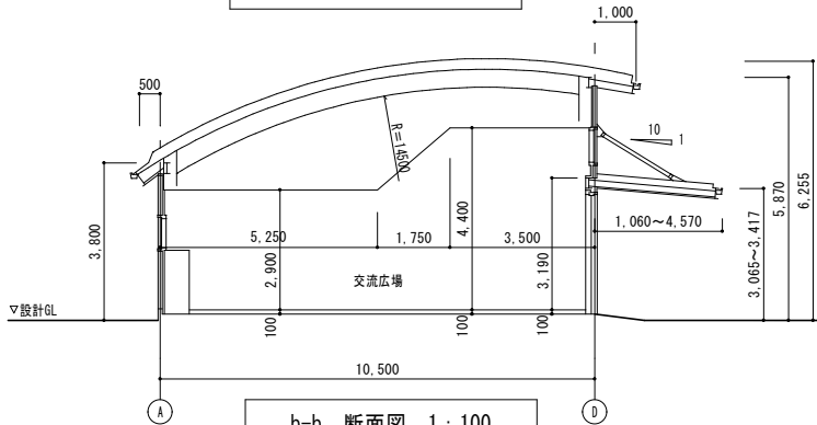
b-b 断面図 1 : 100
