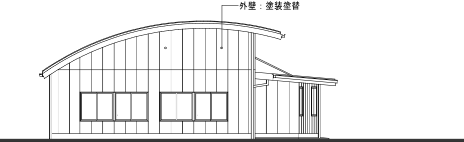
南立面図 1 : 100
