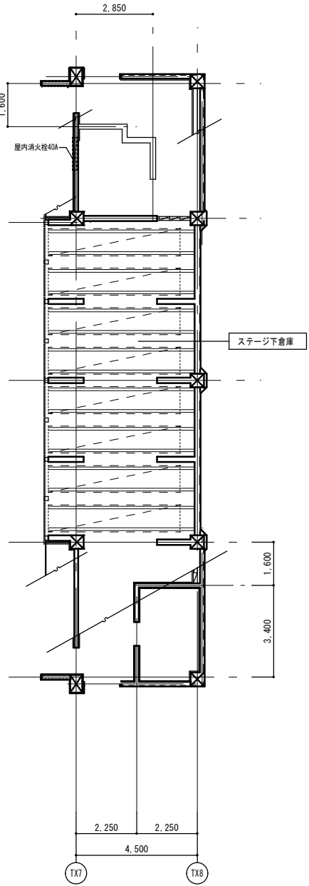
ステージ下平面図 1 : 100
