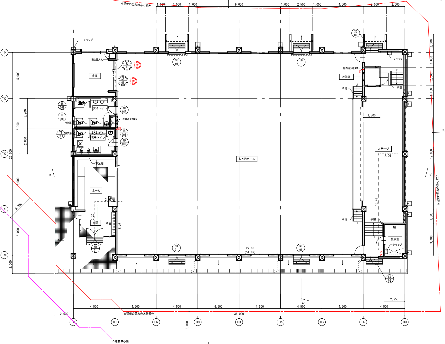
1階平面図 1:100
