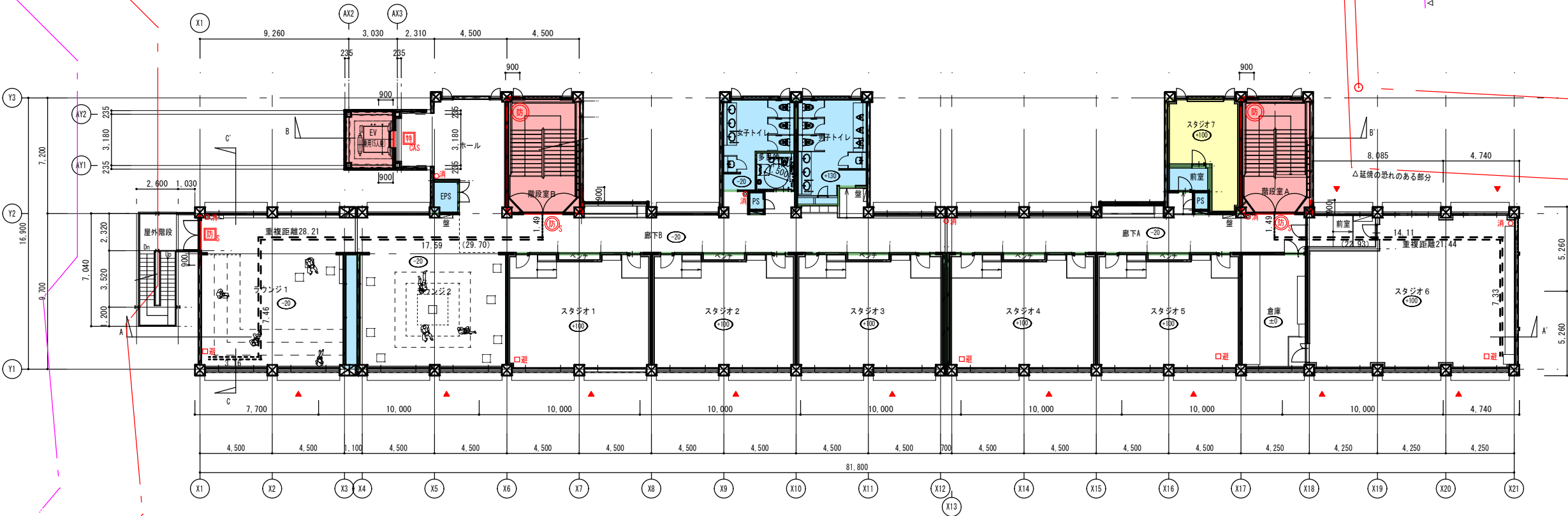
4階平面図 1 : 150
