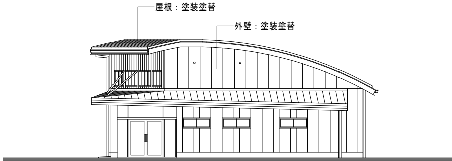
北立面図 1 : 100
