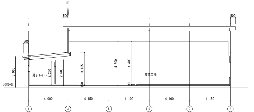
a-a 断面図 1 : 100
