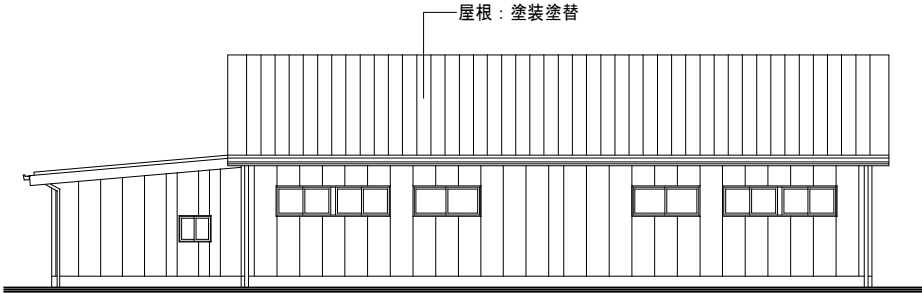
西立面図 1 : 100
