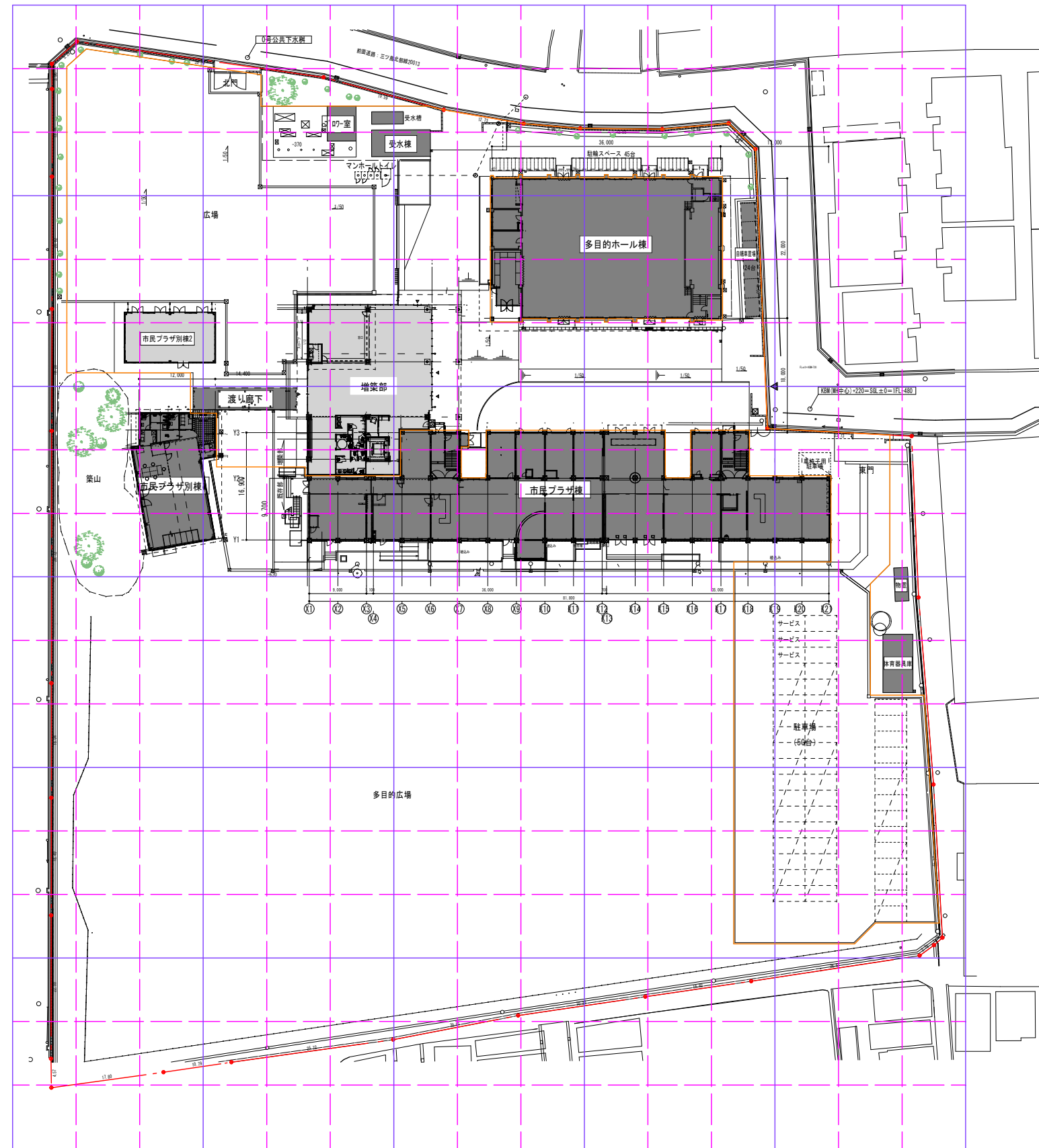
配置図 1 : 300
