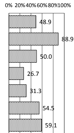
【建物の倒壊】
