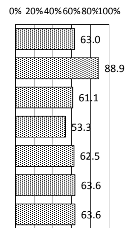
【建物の倒壊】
